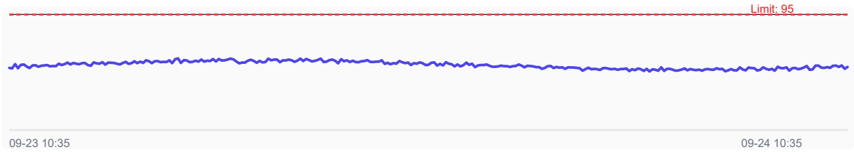
Signal Trend: Bearing_Temp_DE (°C)
